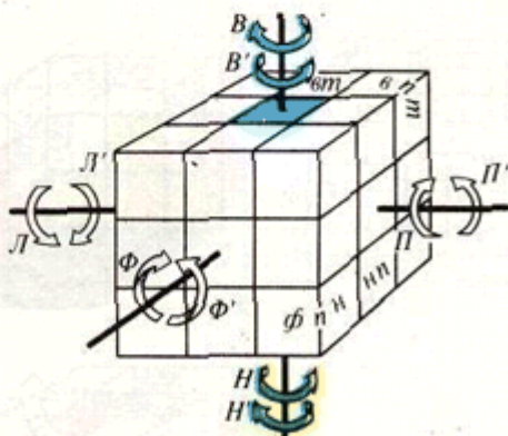
Рис. 0. «Стрелочные» и «буквенные» обозначения поворотов пяти граней (задняя грань нам не понадобится). Например, буква Ф обозначает поворот передней (Фасад) грани на 90^\circ по часовой стрелке, F' — ее поворот на 90^\circ против часовой стрелки, F^2 — ее поворот на 180^\circ . На этом и следующих рисунках незакрашенные грани кубиков — это грани, цвет которых на данном рисунке мы не желаем фиксировать.
