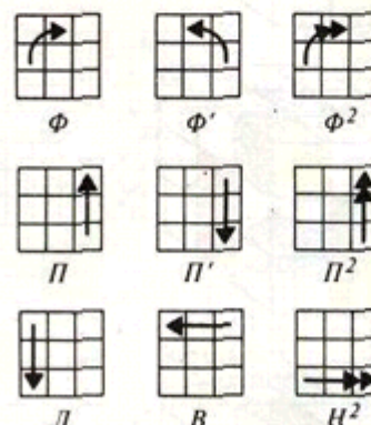
Рис. 0. «Стрелочные» и «буквенные» обозначения поворотов пяти граней (задняя грань нам не понадобится). Например, буква Ф обозначает поворот передней (Фасад) грани на 90^\circ по часовой стрелке, F' — ее поворот на 90^\circ против часовой стрелки, F^2 — ее поворот на 180^\circ . На этом и следующих рисунках незакрашенные грани кубиков — это грани, цвет которых на данном рисунке мы не желаем фиксировать.
