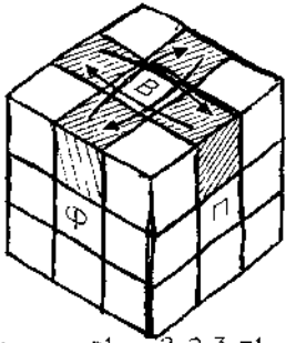
A4 \Phi T^{-1} B (P^2 B^2)^3 B^{-1} T \Phi^{-1} \begin{cases} \delta l \leftrightarrow \delta p \\ \delta \phi \rightarrow \delta \tau \end{cases}
