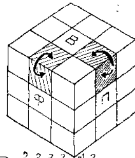
A6 P^2 \Phi P^2 \Phi^{-1} B^2 P \Phi B \Phi^2 \Phi^{-1} \phi \delta \rightarrow \phi \delta
