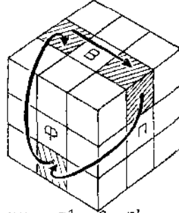
A5 B P^{-1} \Phi^2 P L^{-1} B \begin{cases} \phi H \rightarrow \delta l \rightarrow \delta p \\ \delta \dot{H} \rightarrow \phi H \end{cases}
