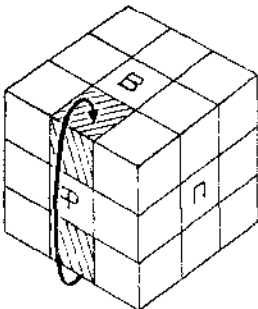
A10 L^{-1} P \Phi^2 L P^{-1} H^2 \phi \dot{H} \rightarrow \phi \delta
